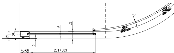
Dušinurkade BLCP4 ja BLCP4 Sabina joonis
