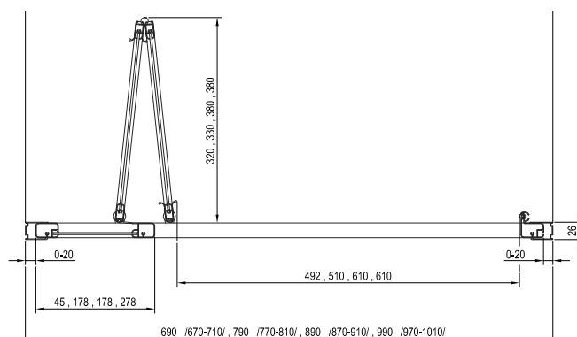
Dušiüste SDZ2-70, SDZ3-80, SDZ3-90, SDZ3-100 joonis
