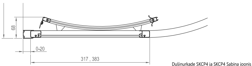
Dušinurkade SKCP4 ja SKCP4 Sabina joonis
